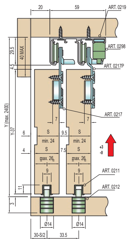
S: ajtólap vastagság (mm) Y: korpusz belmagasság (mm)
