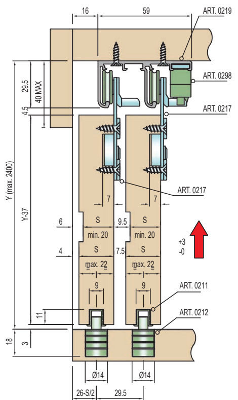
S: ajtólap vastagság (mm) Y: korpusz belmagasság (mm)
