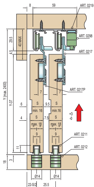
S: ajtólap vastagság (mm) Y: korpusz belmagasság (mm)
